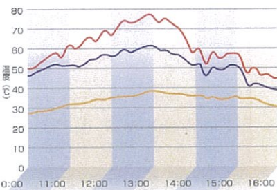
金属BOX屋根面の表面温度比較 クールタイト 汎用屋根用塗料 外気温
